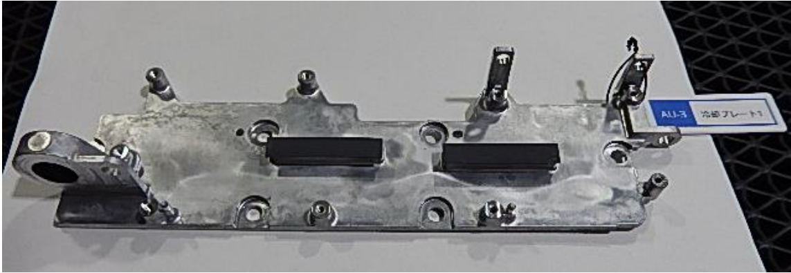
冷却プレート 1
