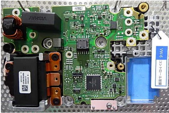
コントロール基板
