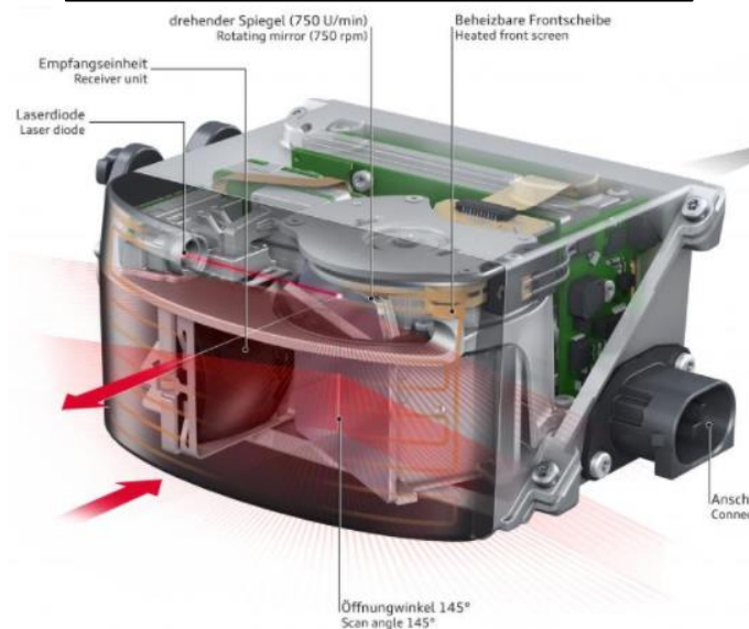
レーザー scanner の内部構造
