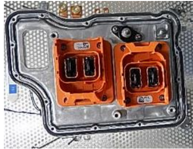
端子台
