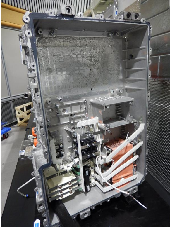
下段ケース
