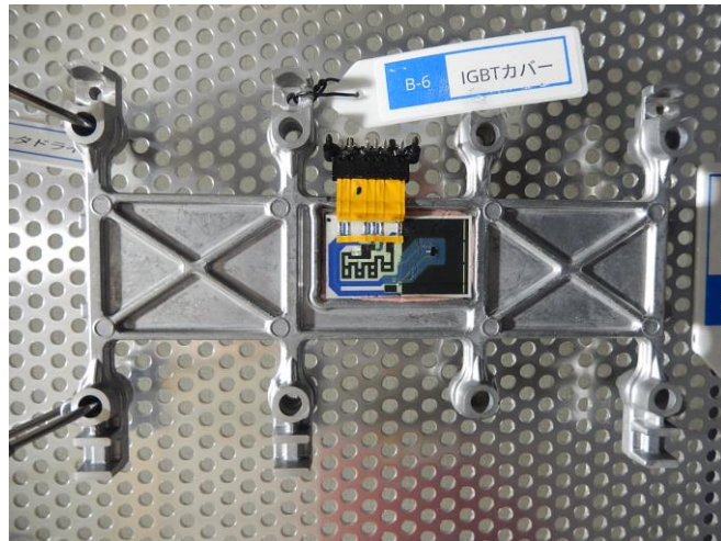
IGBTカバー
